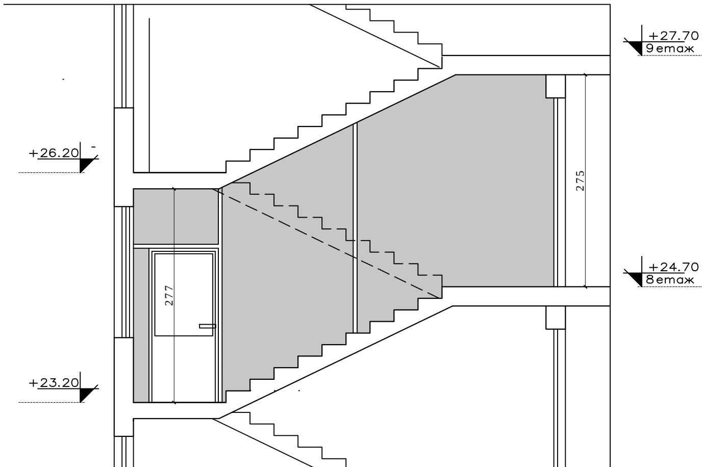
Разрез А—А
