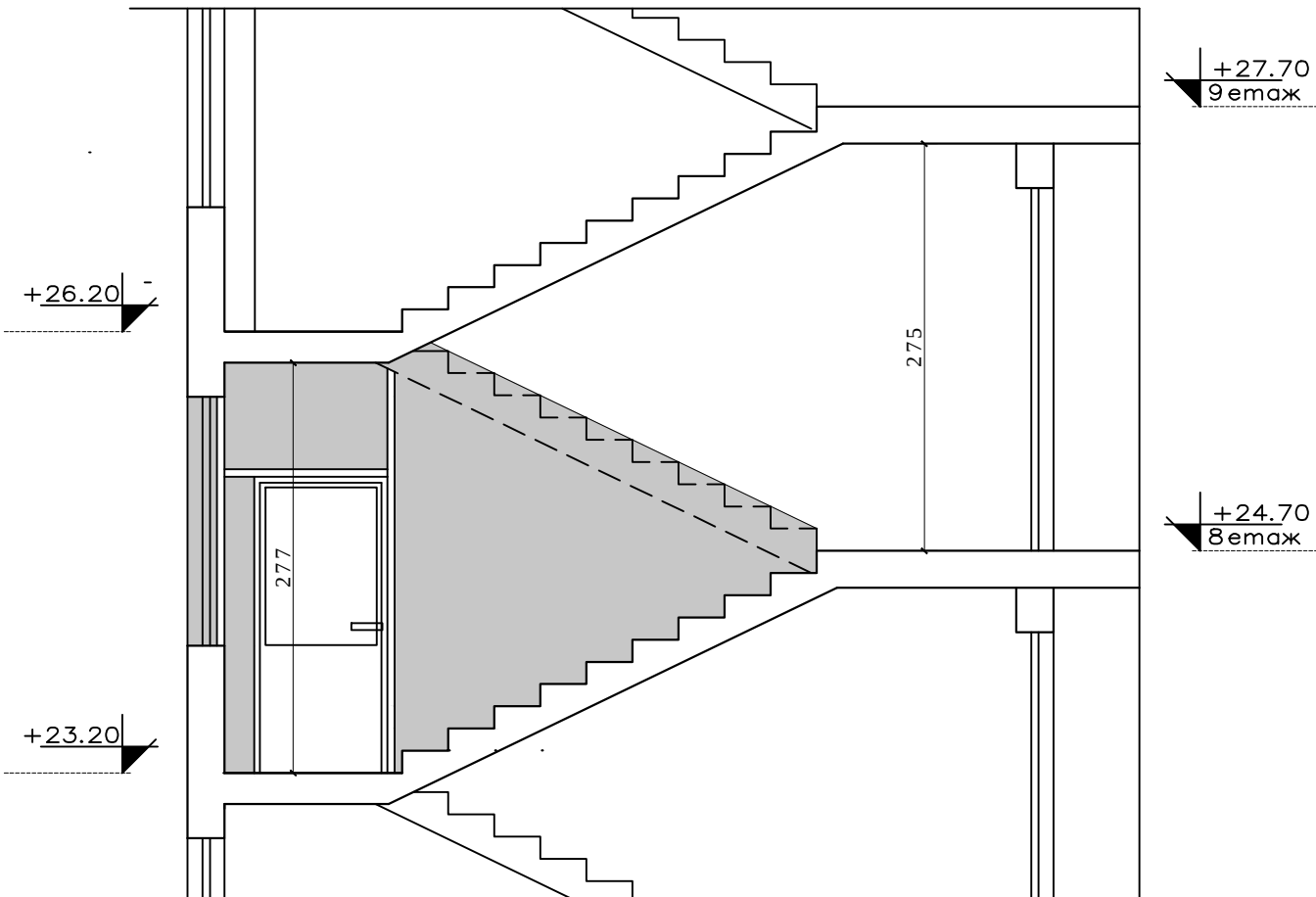
Разрез А—А
