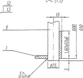
C-C (1:2)
