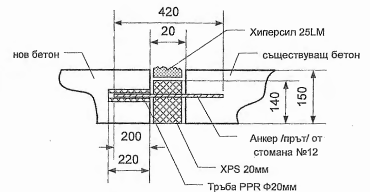
Детайл 2 на нова работна fuga
