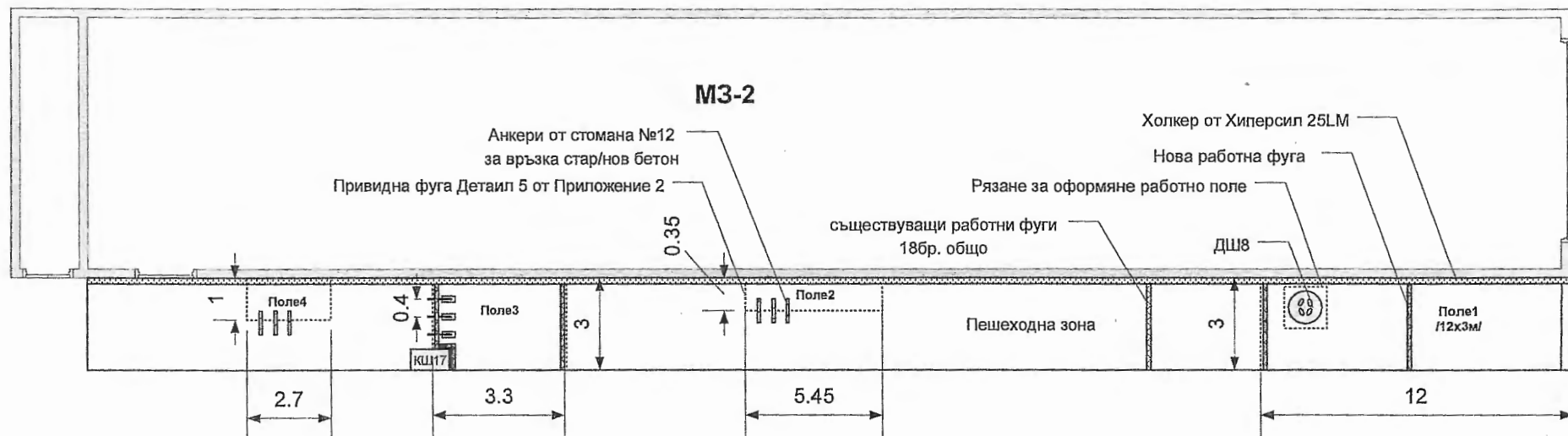
Детайл 2 на нова работна fuga
