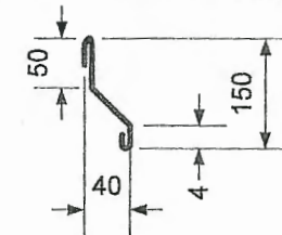
Пола борд запад ЕКЗ ДГС 102
